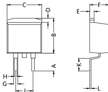
Dimensions TO-263(D 2 PAK)
