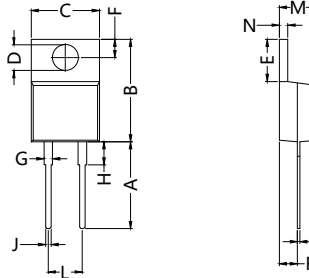
Dimensions TO-220AC
